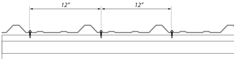
FASTENER PATTERN 12"–12"–12" (over steel purlin)
